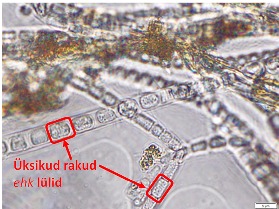
Foto 4. Niitjad rauabakterid 100 kordse suurenduse all vaadatuna (värvimata proov). Fotel on näha rauabakteri silindrikujulised lülid eralduvad ühekaupa limast moodustunud toru otsast ning kanduvad veevooluga piki veetoru edasi kuni leiavad eest takistuse kuhu saab kinnituda. Kui kinnitumine on toimunud saavad rakud hakata poolduma ja uusi niite moodustama.
