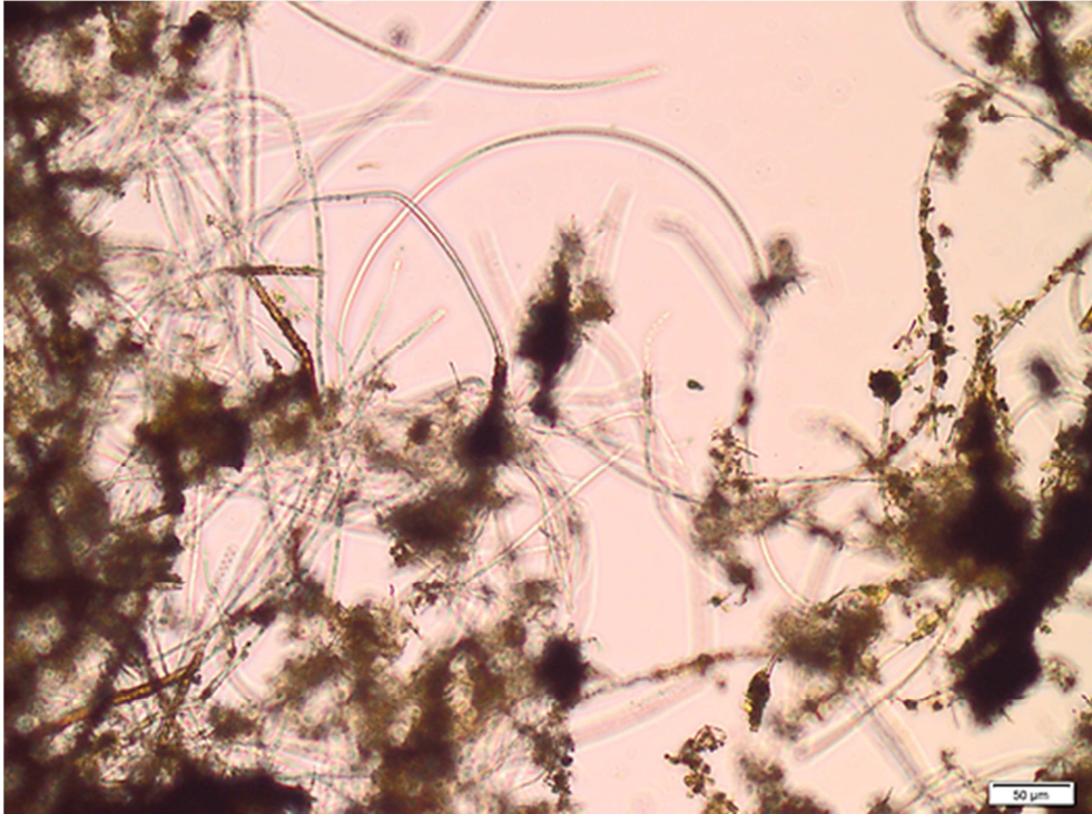
Foto 1. Niitjad rauabakterid. Proov võetud põhjavee torule paigutatud nn mudafiltrist (rauarooostevarvi mass) – amorfse rauasademe vahel on näha läbipaistvad rauabakterite niidid. Suurendus 200 kordama (skaala 50μm, värvimata preparaati).
