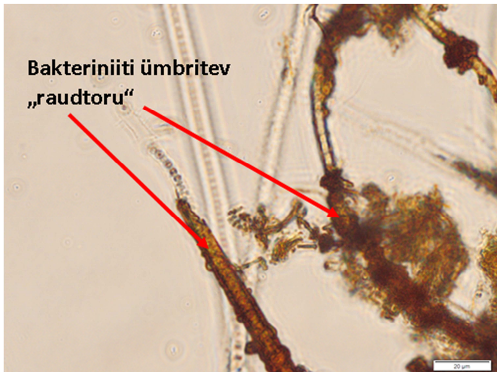
Foto 3. Proovis olevad rauabakterid kasvatavad enda ümber amorfsest kolmevalentsest rauast kihi - toru (näidatud punase noolega; värvimata proov).
