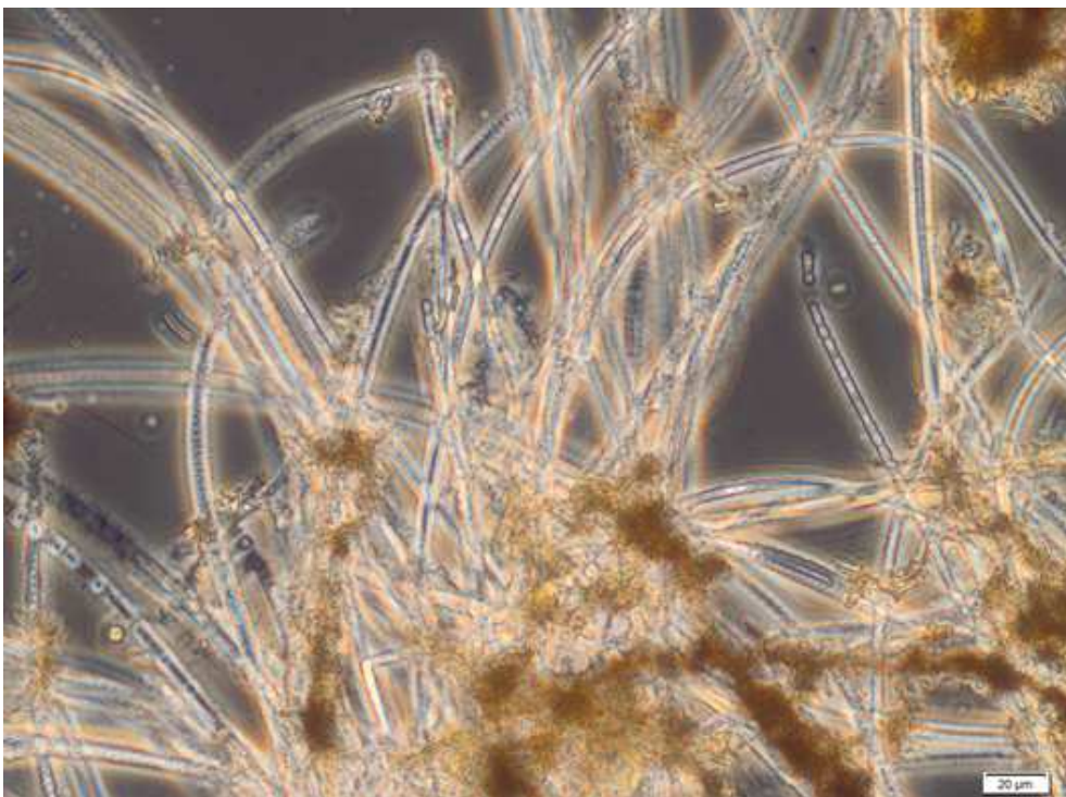
Foto 2. Samad rauabakterid, mis fotol 1 , suurendus 400 korda (skaala 20μm, värvimata preparaati). Fotol on näha, et rauasade ümbritseb rauabakterite niite, mis tõestab, et rauasete on tekkinud bakterite elutegevuse tulemusena.
